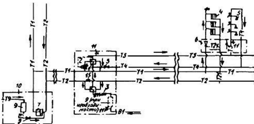
Рис.1. Схема закрытой системы теплоснабжения
