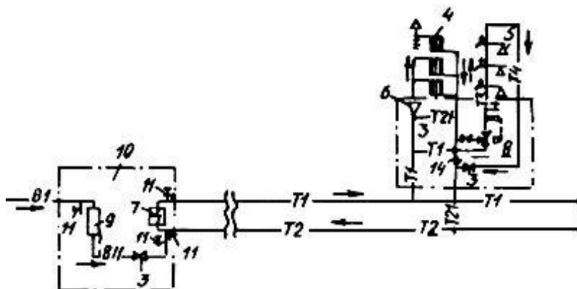
Рис.2. Схема открытой системы теплоснабжения
