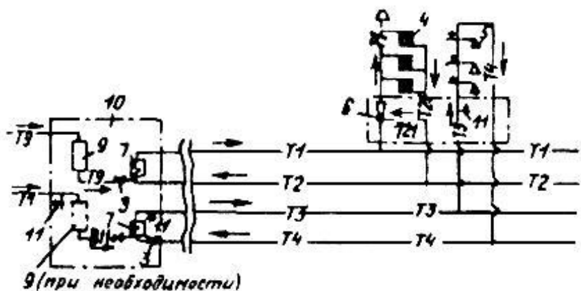
Рис.3. Схема теплоснабжения с отдельными сетями горячего водоснабжения
